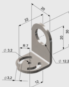
Equerre ajustable sur 1 axe (ACCTFB)
