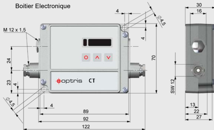
Boîtier Electronique
