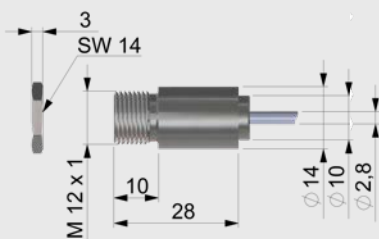
Tête de mesure
