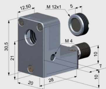
Buse de soufflage laminaire, en option optique CF intégrée (ACCTAPLCFHT)
